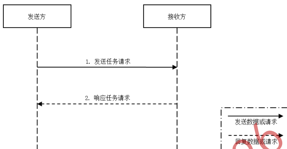
图 9 任务请求发送接口通信流程
