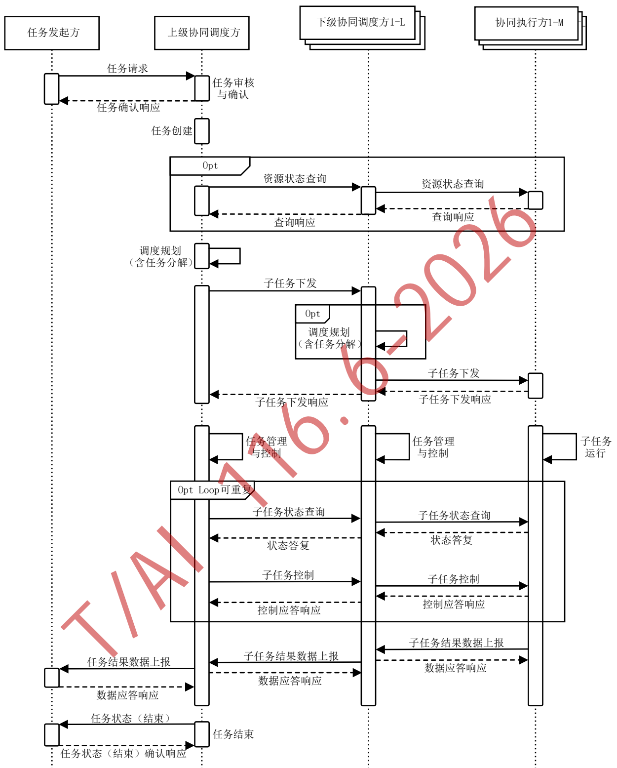
图 B.2 级联协同模式下自上而下发起任务时的协同工作交互流程
